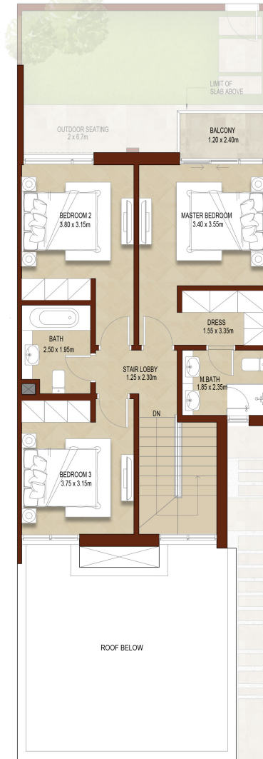
FIRST LEVEL الطابق الأول
