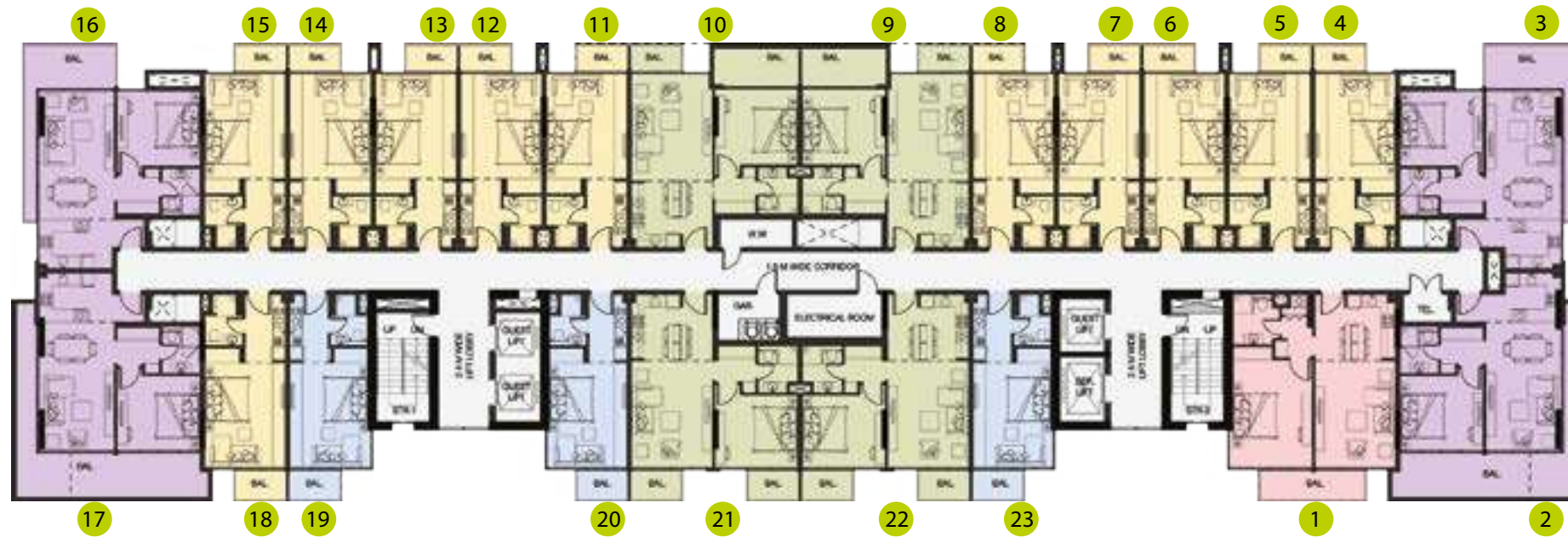
الطوابق النموذجية من السادس إلى التاسع 6th to 9th Typical Floors
